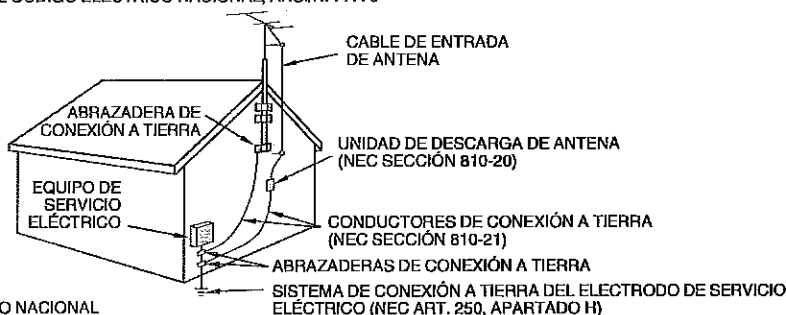
EJEMPLO DE CONEXIÓN A TIERRA DE LA ANTENA SEGÚN EL CÓDIGO ELÉCTRICO NACIONAL, ANSI/NFPA 70
